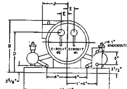
END ELEVATION
